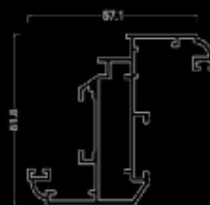
پروفیل لنگه
