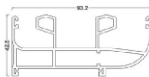
پروفیل فریم سری 62
