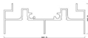
جنب پایه دار ST
