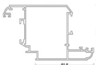
پروفیل لنگه
