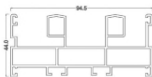
پروفیل فریم سری 94
