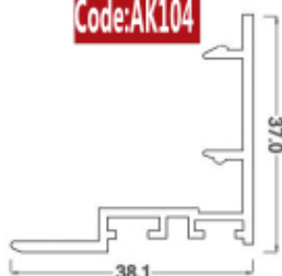
درپوش
