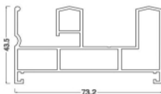
پروفیل فریم سری 73
