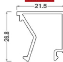
زهوار تک جداره
