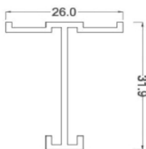
سپری سقفی 4
