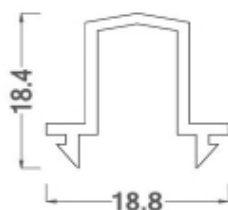
پروفیل وسط چهار لنگه
