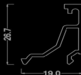
زهوار دوجداره
