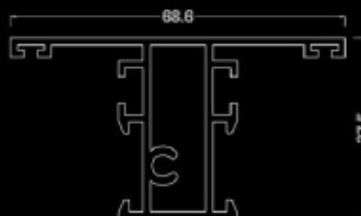
پروفیل سپری
