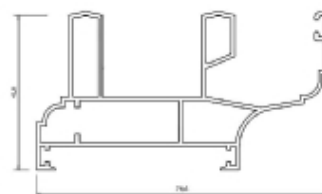
پروفیل فریم سری 55
