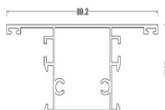
پروفیل سپری
