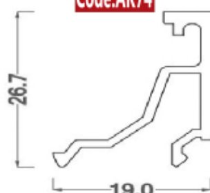
زهوار دو جداره
