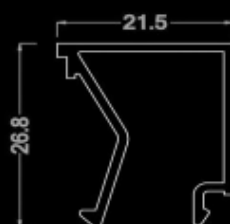
زهوار تک جداره
